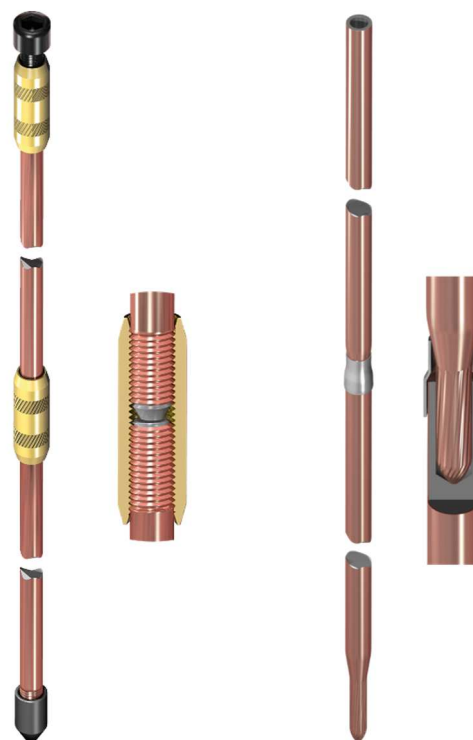
Rys. 1. Uziomy pionowe pomiedziowane: a) gwintowany; b) kuty z powłoką Cu 250 \mu\text{m}
