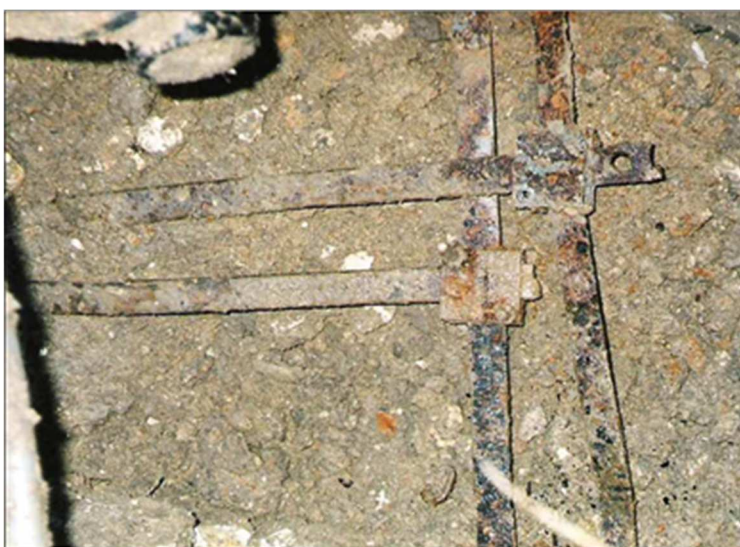
Rys. 4. Skorodowana bednarka ocynkowana po 12 latach eksploatacji
