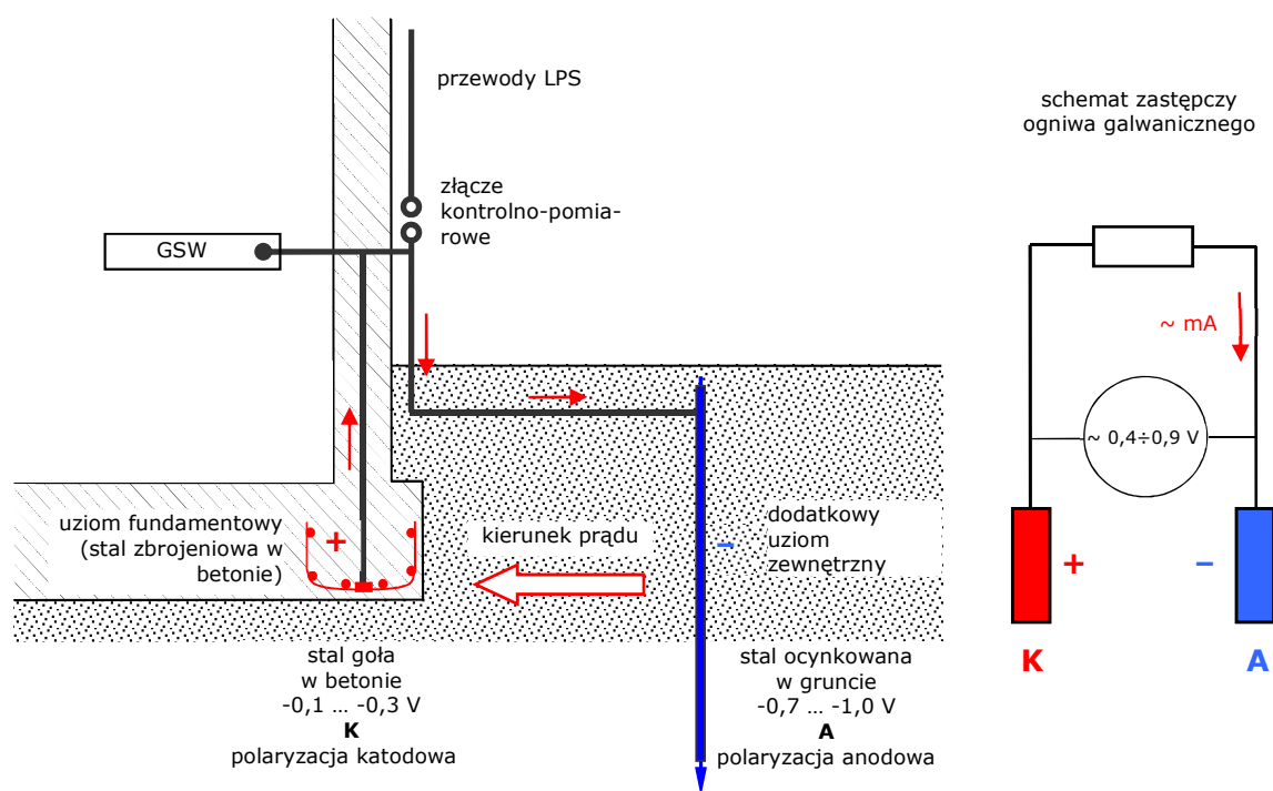
Rys. 5. Zagrożenie korozją elektrochemiczną w wyniku połączenia uziomu fundamentowego i uziomu zewnętrznego ze stali ocynkowanej
