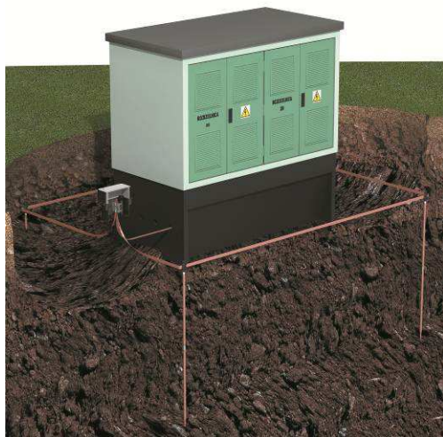
Rys. 3. Uziemienie stacji transformatorowej
